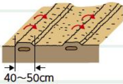
図2 畑の準備2
