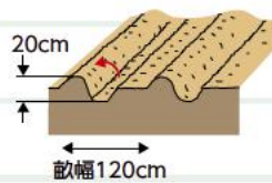
図1 畑の準備1
