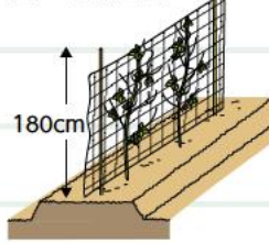
図4 支柱立て
