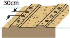
図3 種まき
